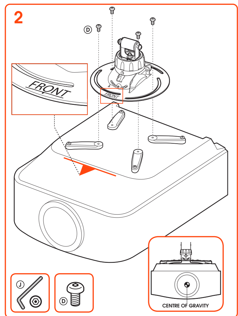
PPC 2500
