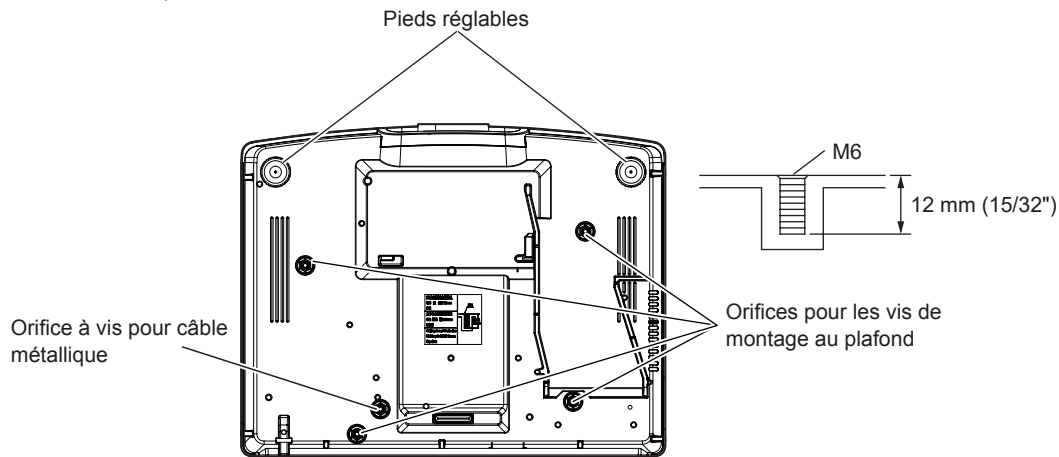
Positions des orifices pour les vis de montage au plafond et des pieds réglables
